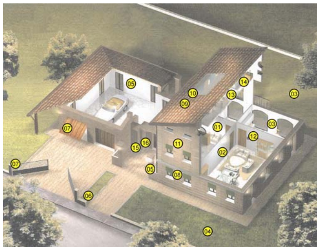
Slika 3. – Prikaz zasnove EIB instalacije
